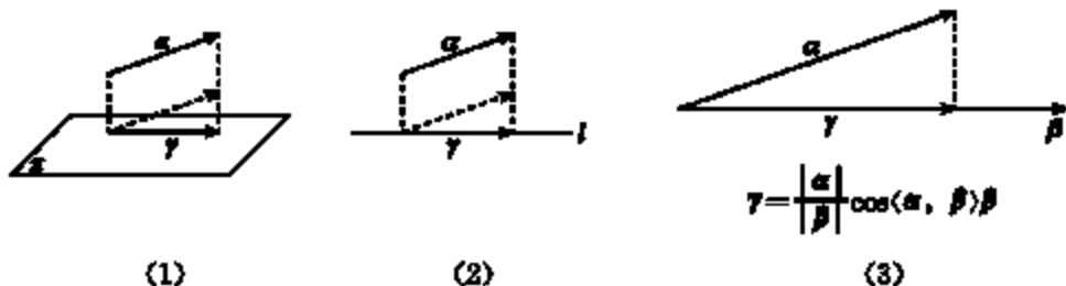
图9 向量投影
