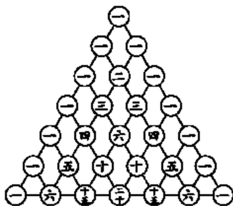
图 12 杨辉三角
